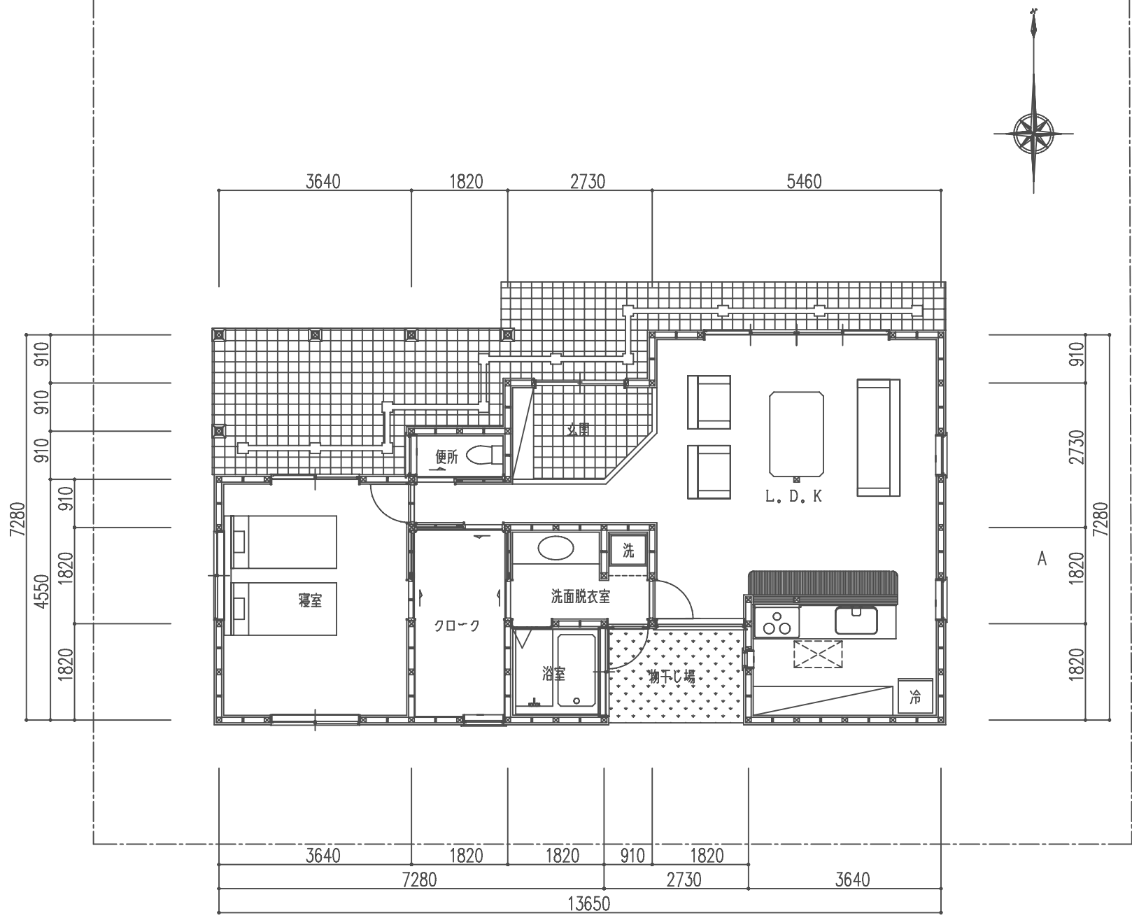
1階平面図 1:100
