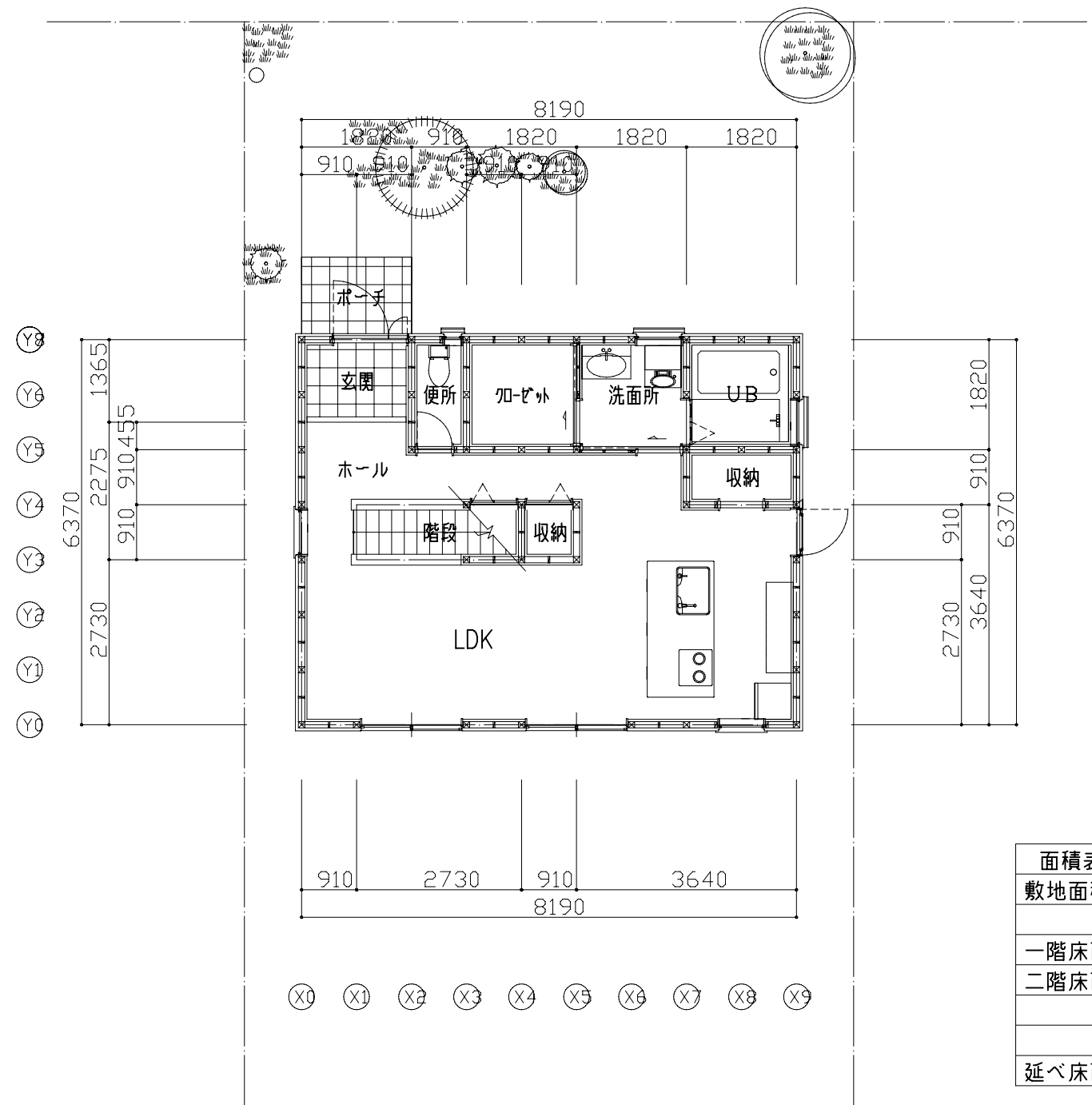
1階平面図 1:100
